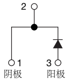
2L TO-220AC
