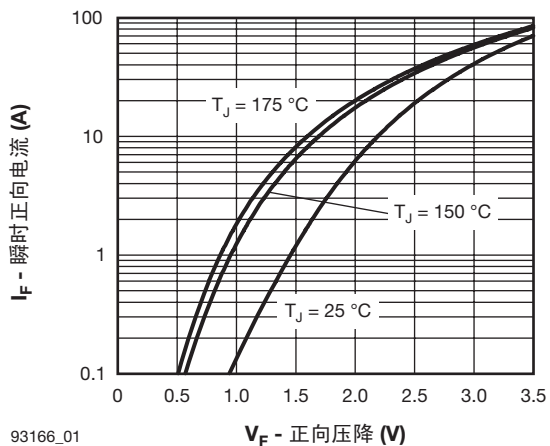
图 1. 典型正向压降特性图
