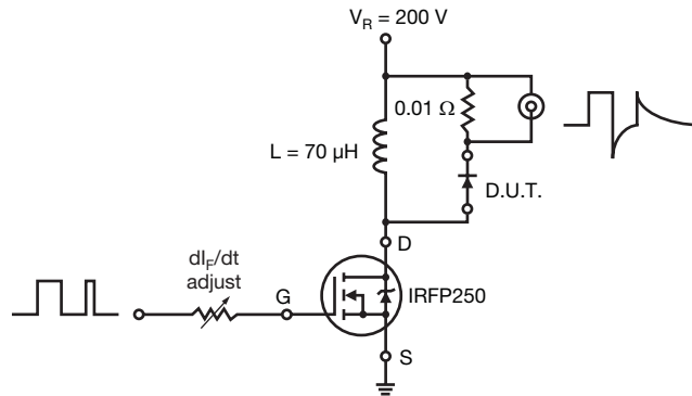
图 11. 反向恢复参数测试电路
