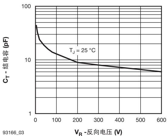
图 3. 典型结电容和反向电压关系图
