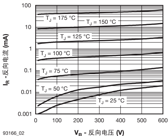
图 2. 反向电流与反向电压典型值
