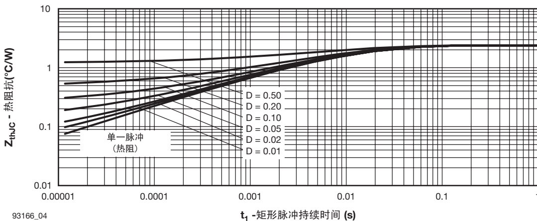
图 4. 最大热阻抗 Z_{thJC} 特性图 (TO-220)
