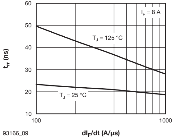
图 9. 典型反向恢复时间和 dI_F/dt 关系图
